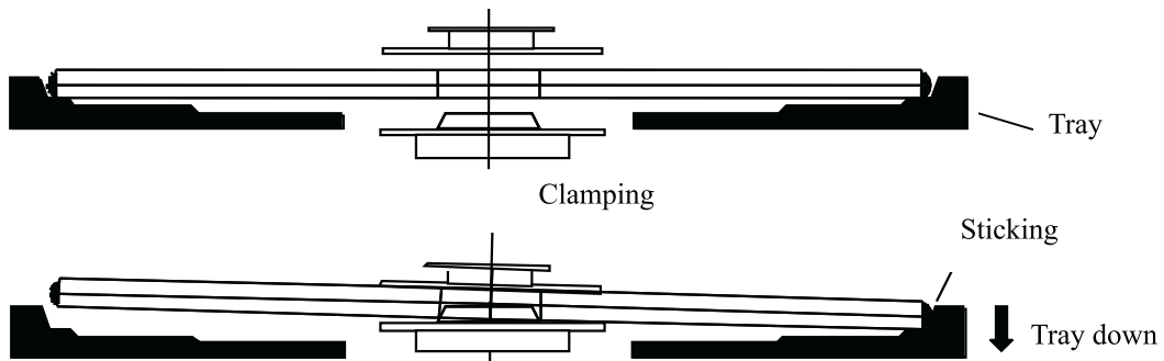
Figure N.3 - Burr
